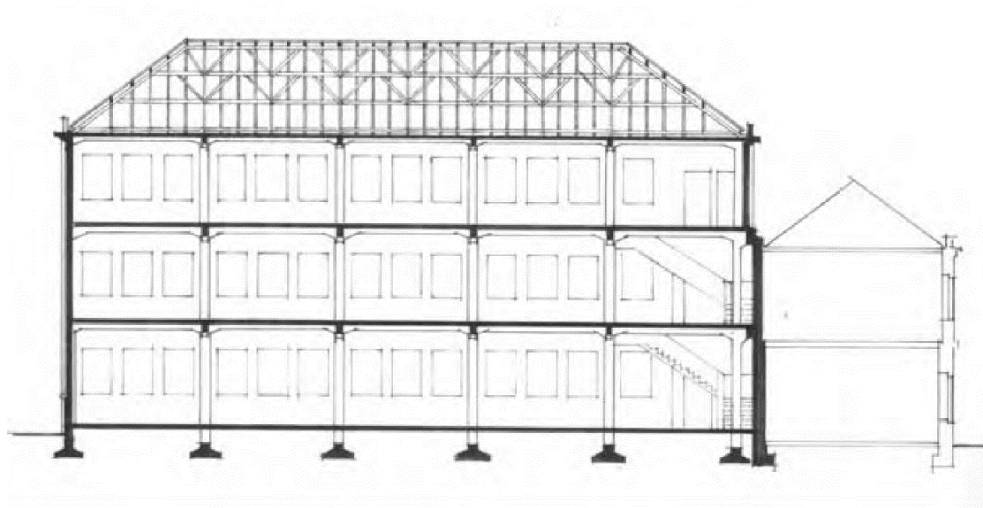
Imagem 2 - Planta longitudinal do prédio da Neugebauer inaugurado em 1904
