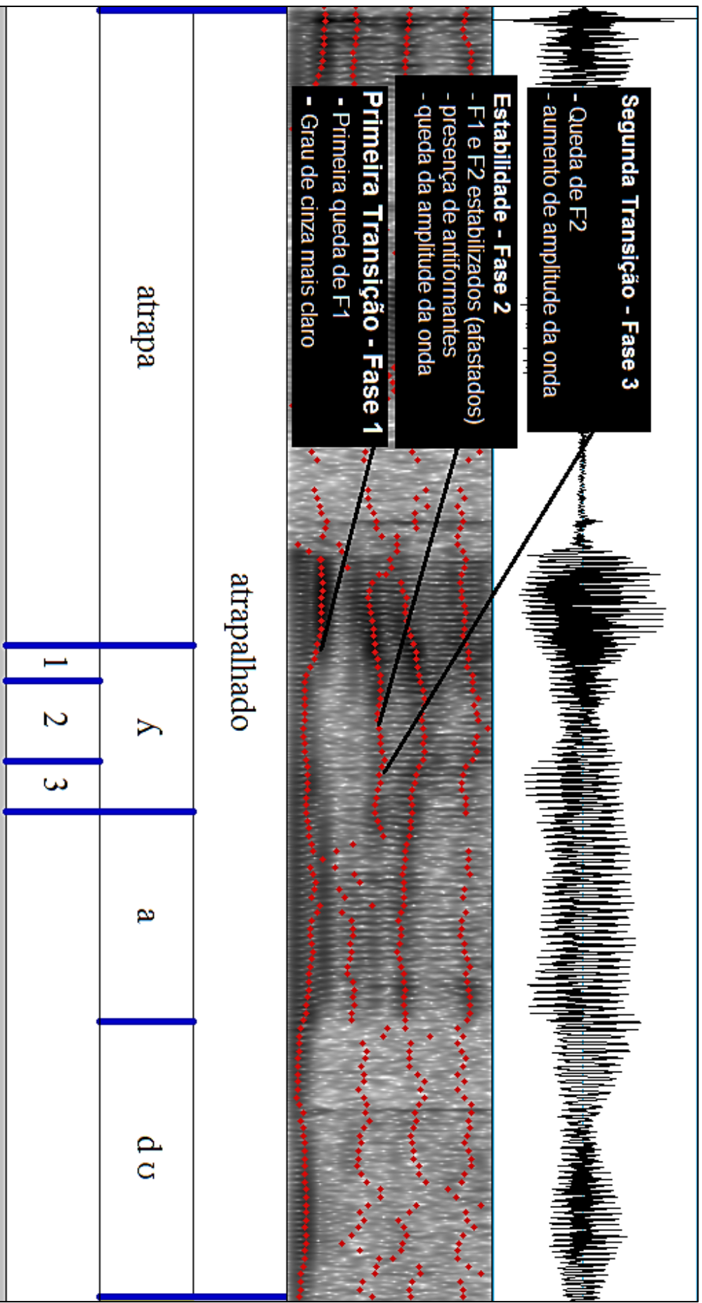
Figura 17. Fases acústico-articulatórias de [ʎ] – Informante feminino, 22 anos.
