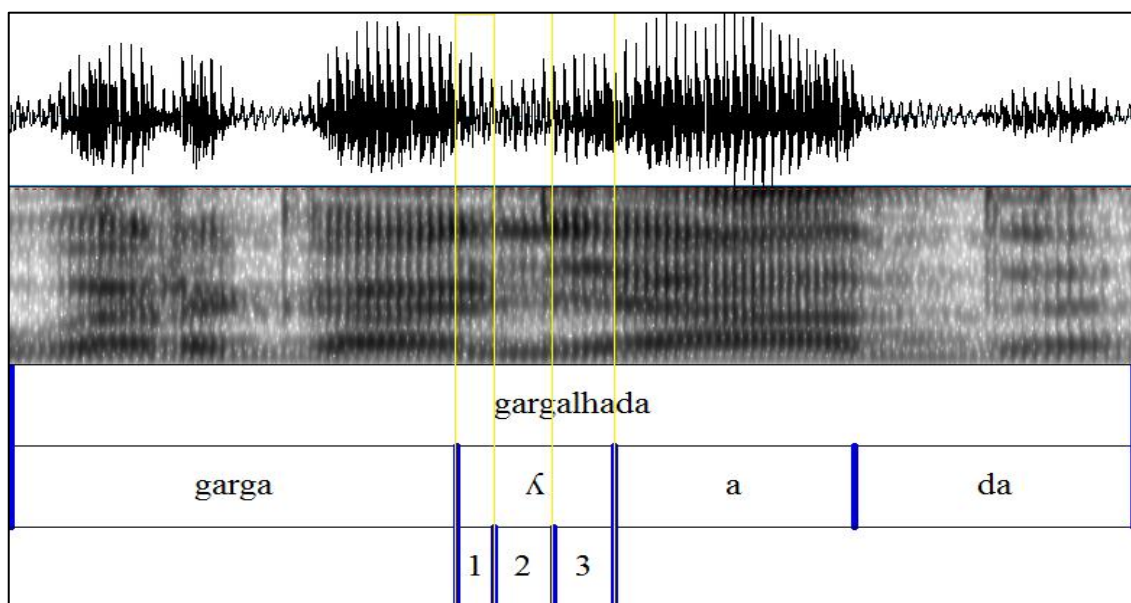
Figura 16: Exemplo das anotações nos dados acústicos – informante masculino, 22 anos.
