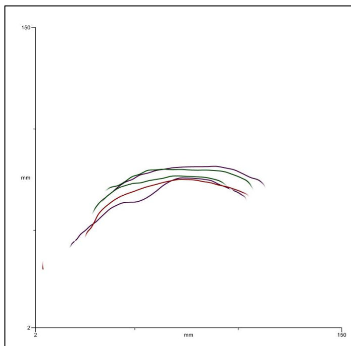
Gráfico 13: Curvas de língua no ponto médio de [ʎ] para as duas produções de “atrapalhado”, “palhaço” e “gargalhada”. Legenda: linhas em verde, o ponto médio da fase central das duas produções de “atrapalhado”; linhas em vermelho, o ponto médio da fase central das duas produções de “palhaço”; linhas em roxo, o ponto médio da fase central das duas produções de “gargalhada” – Informante U.I.C.
