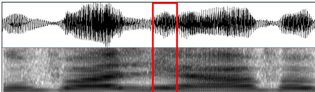
Figura 28: Espectro da palavra “valhava”, com destaque para a Fase 3. Informante V. (ouvinte, feminino, 22 anos)
