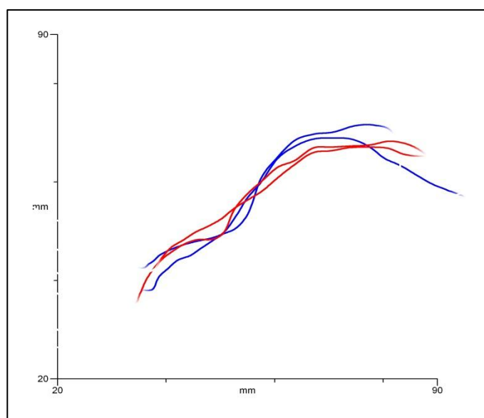
Gráfico 14: Curvas de língua no ponto média da fase central da lateral palatal em palavras foneticamente semelhantes. Legenda: linhas em azul, o ponto médio da fase central das duas produções de “valioso”; linhas em vermelho, ponto médio da fase central das duas produções de “trabalhoso”. Informante V
