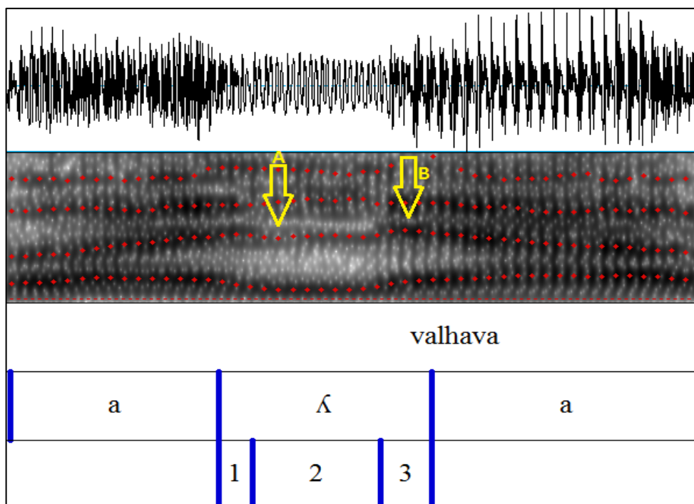
Figura 20: Imagem espectrográfica ampliada do logatoma “valháva”. Em “A” os antifomantes e em “B” o segundo formante. - Sujeito L.
