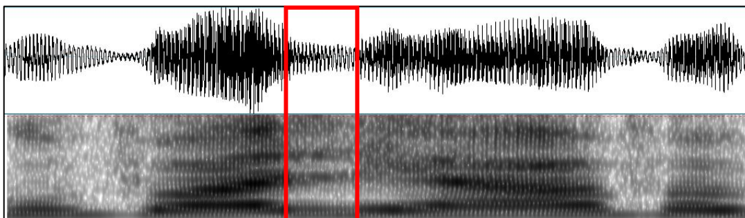
Figura 26: Espectro da palavra “valhava”, com destaque para a Fase 2. Informante V. (ouvinte, feminino, 22 anos)
