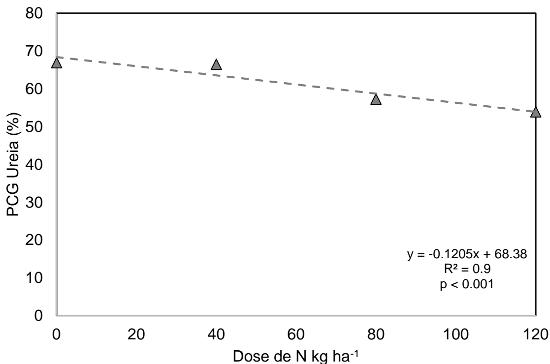
Figura 13. Primeira contagem de germinação de sementes de trigo no teste de germinação, produzidas com diferentes doses de nitrogênio suplementadas com ureia.
