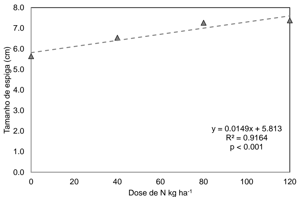
Figura 5. Tamanho de espigas de trigo, sob diferentes doses de nitrogênio.
