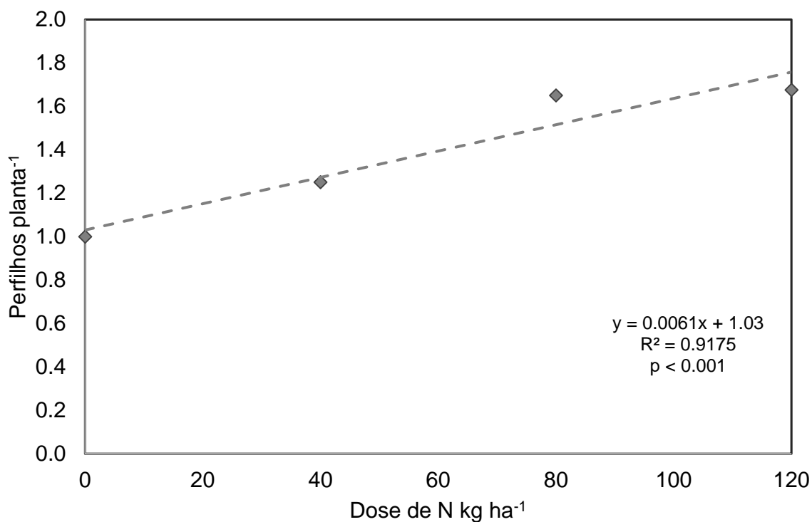
Figura 3. Número de perfilhos por planta de trigo, sob diferentes doses de nitrogênio.
