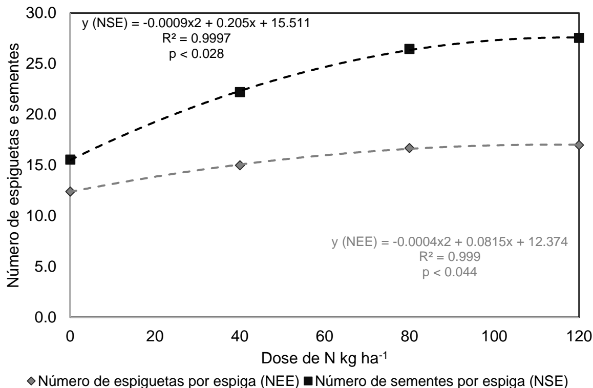
Figura 6. Número de sementes por espiga (NSE) e número de espiguetas por espiga (NEE) de trigo, sob diferentes doses de nitrogênio.
