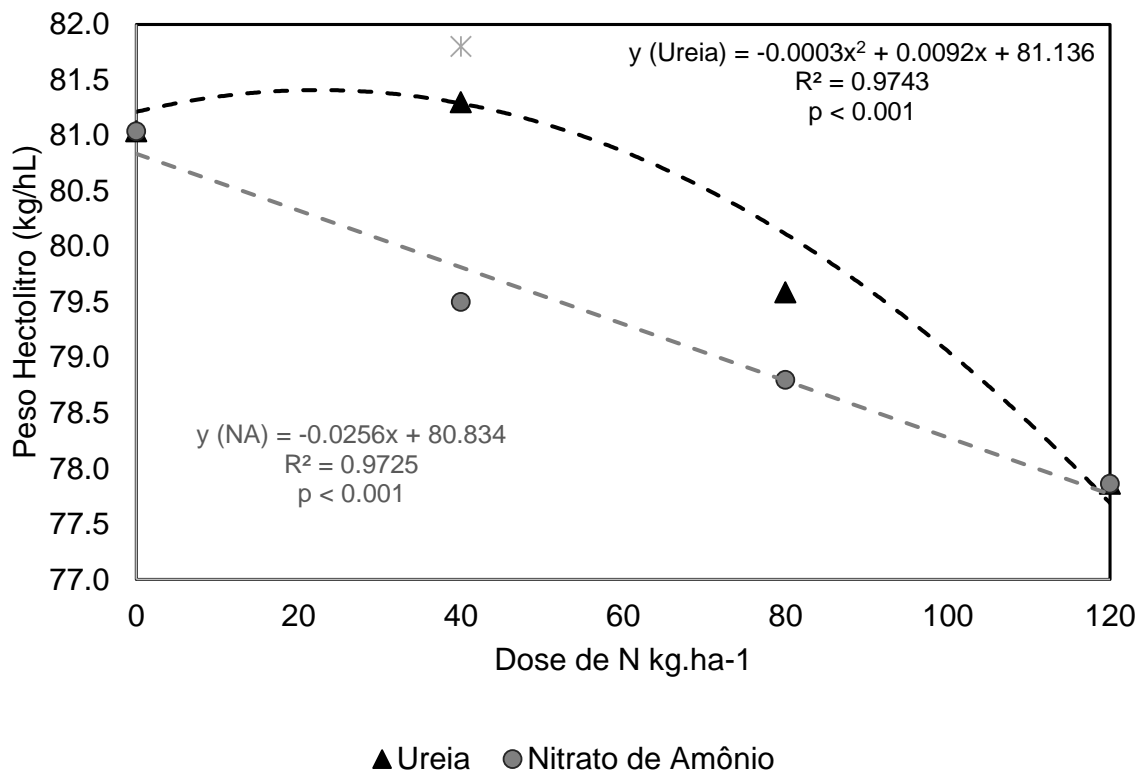
Figura 10. Peso hectolitro de trigo, sob diferentes doses de nitrogênio suplementadas por ureia e nitrato de amônio. Asteriscos na parte superior do gráfico representam diferenças significativas entre fonte de N dentro de cada dose.
