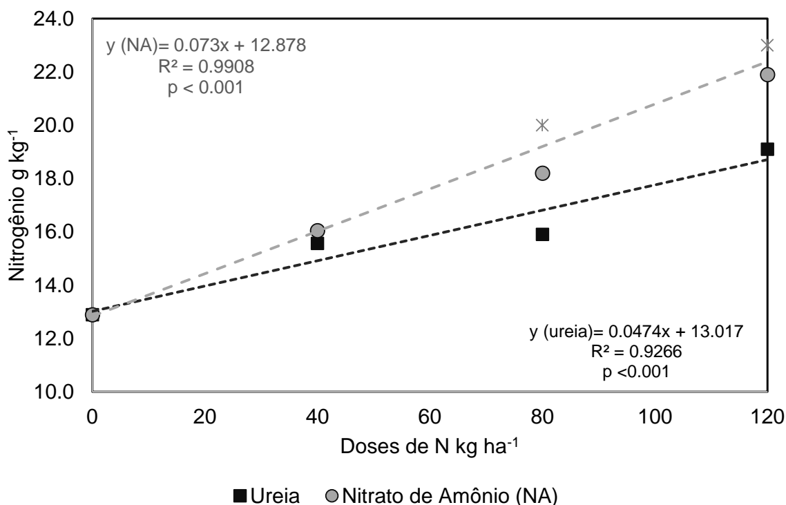
Figura 17. Teor de nitrogênio em sementes de trigo, produzidas com diferentes doses de nitrogênio suplementadas por ureia e nitrato de amônio. Asteriscos na parte superior do gráfico representam diferenças significativas entre fonte de N dentro de cada dose.
