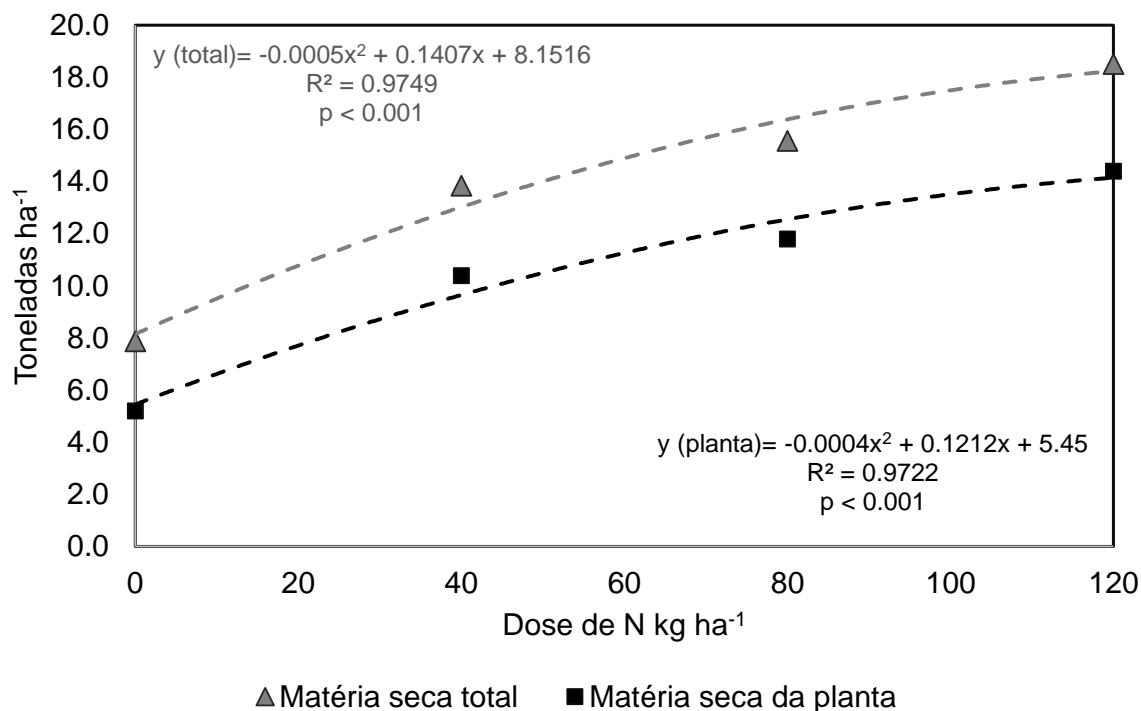
Figura 8. Matéria seca total e de planta de trigo, sob diferentes doses de nitrogênio.
