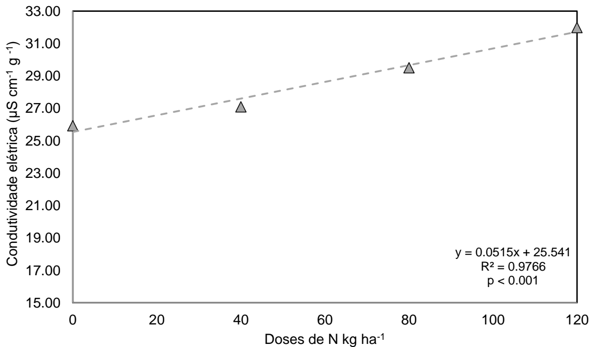
Figura 16. Resultado do teste de condutividade elétrica em sementes de trigo, produzidas com diferentes doses de nitrogênio suplementadas por ureia e nitrato de amônio.
