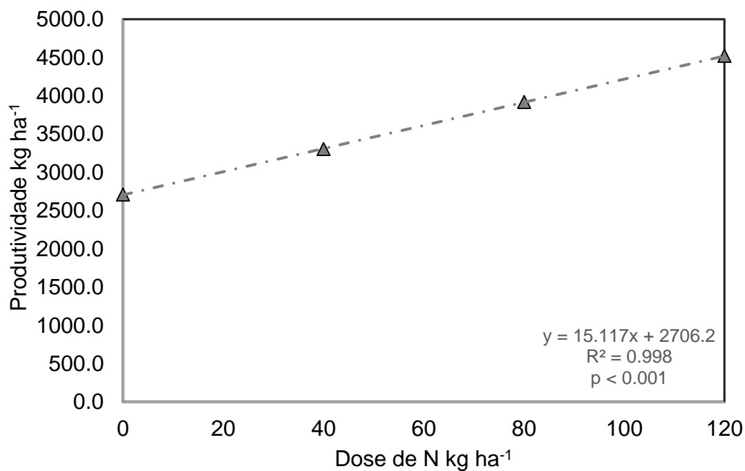
Figura 9. Produtividade de sementes de trigo sob doses de nitrogênio na forma de ureia e nitrato de amônio.
