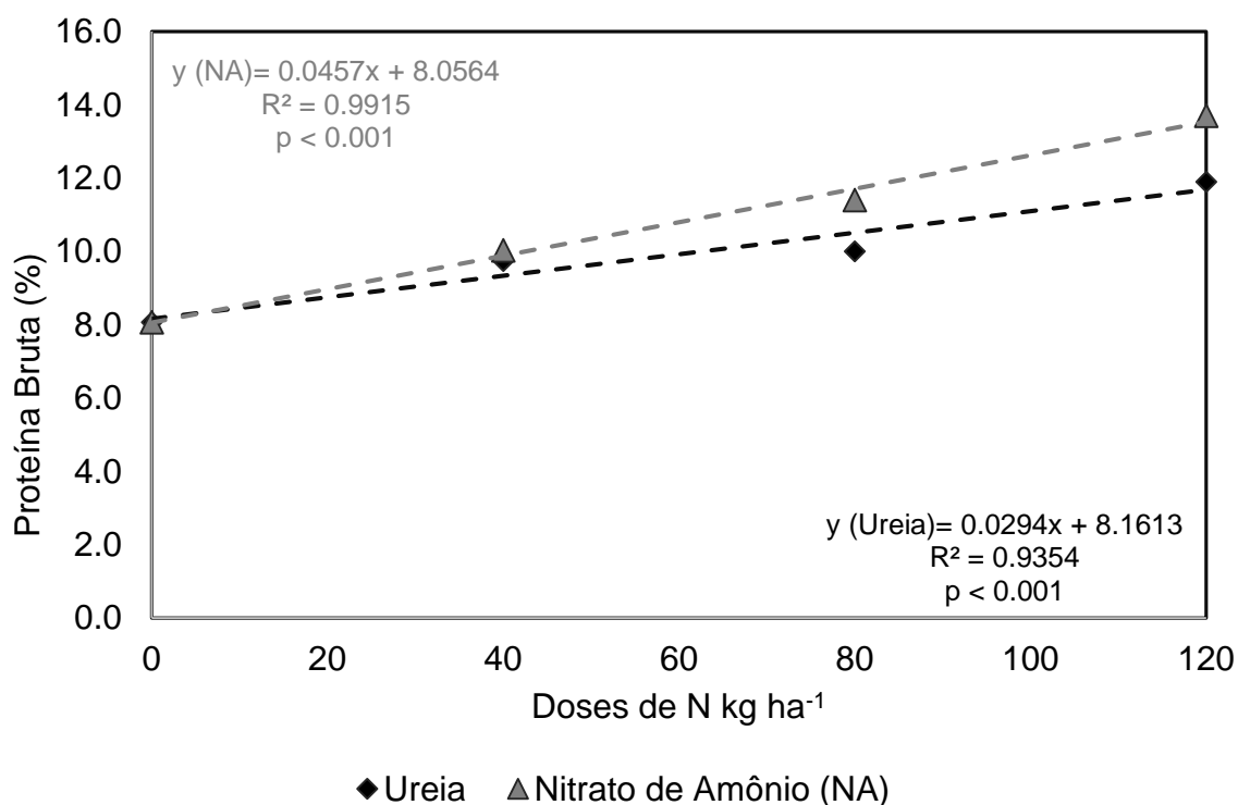
Figura 11. Teor de proteína bruta em trigo, sob diferentes doses de nitrogênio suplementadas por ureia e nitrato de amônio.
