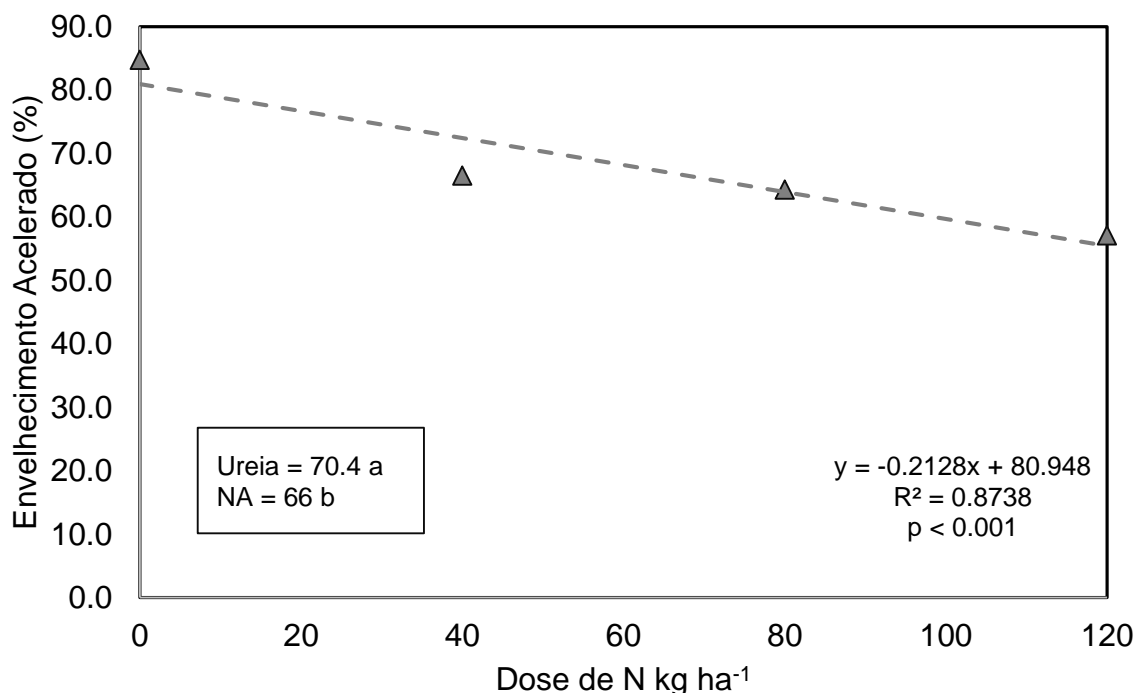
Figura 15. Percentagem de germinação de sementes de trigo no teste de envelhecimento acelerado, produzidas com diferentes doses de nitrogênio suplementadas por ureia e nitrato de amônio.
