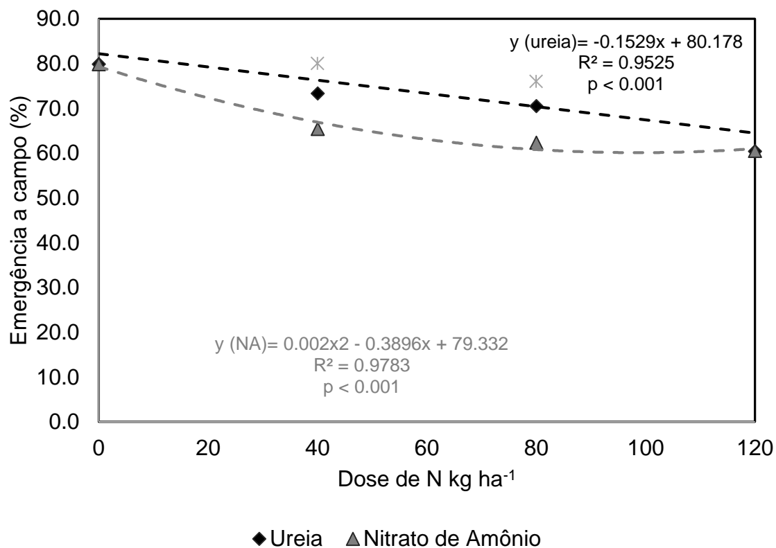
Figura 14. Percentagem de germinação de sementes de trigo no teste de emergência a campo, produzidas com diferentes doses de nitrogênio suplementadas por ureia e nitrato de amônio. Asteriscos na parte superior do gráfico representam diferenças significativas entre fonte de N dentro de cada dose.
