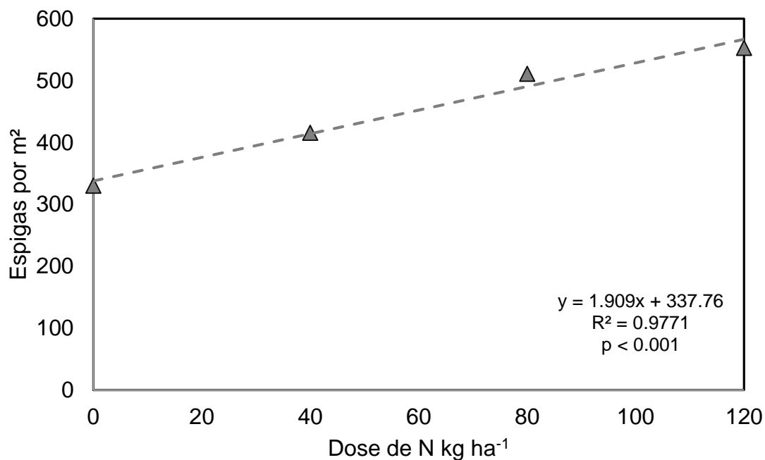
Figura 7. Número de espigas de trigo por metro quadrado de trigo, sob diferentes doses de nitrogênio.
