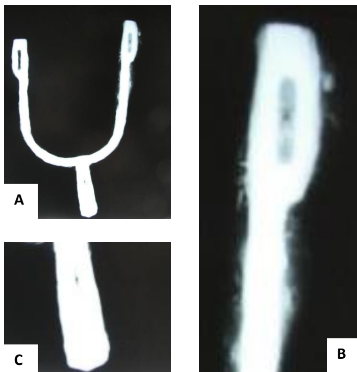
Figura 37. Radiografia de uma espora de ferro dos inícios do século XIX. (A. Imagem radiográfica completa; B. detalhe de um dos extremos ilustrando a abertura e toda a superfície coberta por concreções; C. detalhe da base mostrando a área de inserção da estrela). Fonte: Susana dos Santos Dode.
