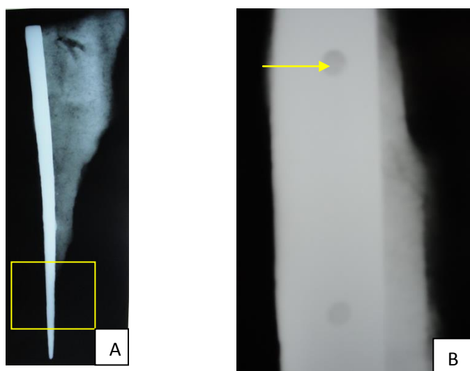
Figura 38. A. Radiografia de um artefato extraído em bloco de um campo de batalha. B. Detalhe de uma seção, mostrando os orifícios que auxiliaram na sua identificação como parte de uma ferramenta de trabalho.
