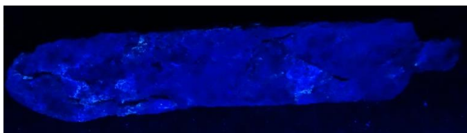
Figura 41. Exame de fluorescência evidenciando áreas de diferentes níveis de oxidação em um artefato arqueológico metálico do século XVIII. Fonte: Susana dos Santos Dode.
