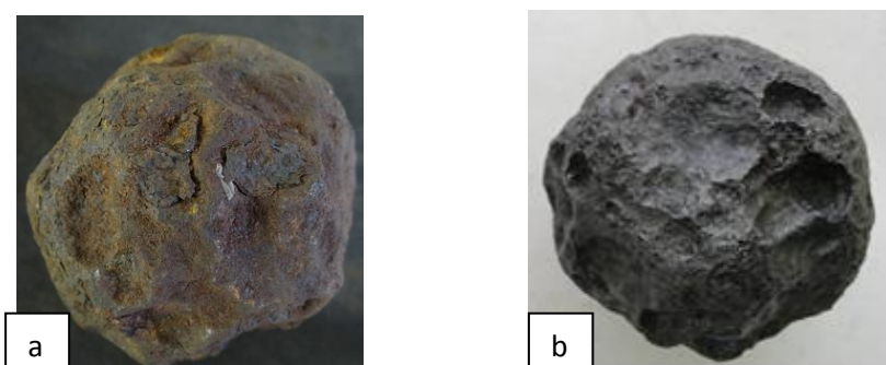
Figura 77 a e b - Bala rasa de canhão antes (a) e depois (b) do tratamento de conservação curativa. Fonte: acervo fotográfico do LÂMINA
