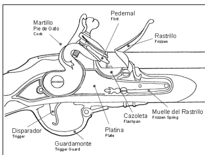
Figura 13. Esquema do sistema mecânico que compõe um fuzil de pederneira. Fonte: https://armasonline.org/armas-on-line/as-armas-do-brasil-na-guerra-do-paraguai/
