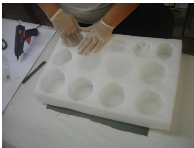
Figura 52. Confecção de embalagens com etaphoam .
