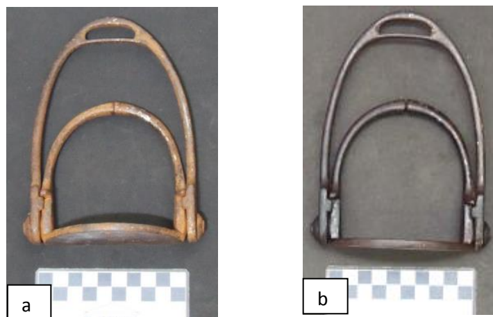
Figura 78 a e b – estribo de balancin antes (a) e depois (b) da aplicação dos tratamentos de conservação curativa.
