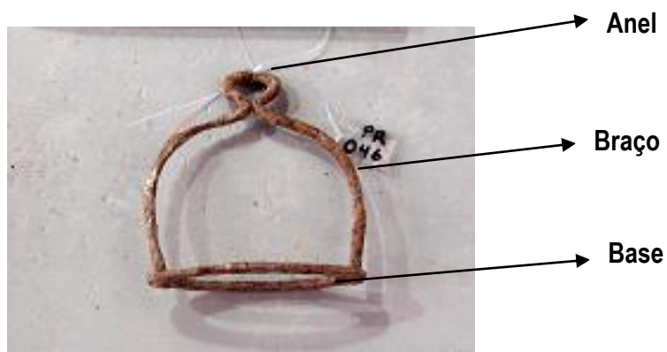
Figura 28. Partes que compõem um estribo de ferro do século XIX. Fonte: Susana dos Santos Dode.
