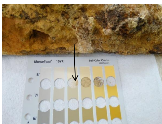
Figura 34. Comparação da cor da concreção com a Carta Mansell de solos. Fonte: Susana dos Santos Dode.
