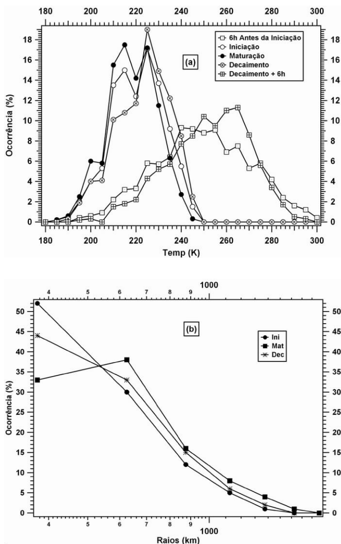
Figura 1: Histogramas da temperatura de brilho infravermelho (Tir) das PC (a) seis horas antes da iniciação (I06), na iniciação (Ini), maturação ou máxima extensão de área (Mat), decaimento (Dec) e seis horas após a dissipação (D06) e histograma dos raios efetivos das PC nas diferentes fases do ciclo de vida (b).
