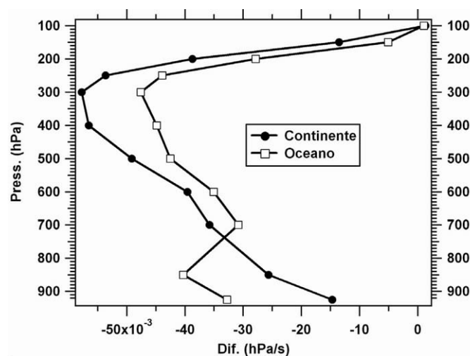
Figura 5: Perfis verticais de omega na presença de perturbações convectivas na região equatorial sobre o continente e o oceano. Unidade (hPa/s).
