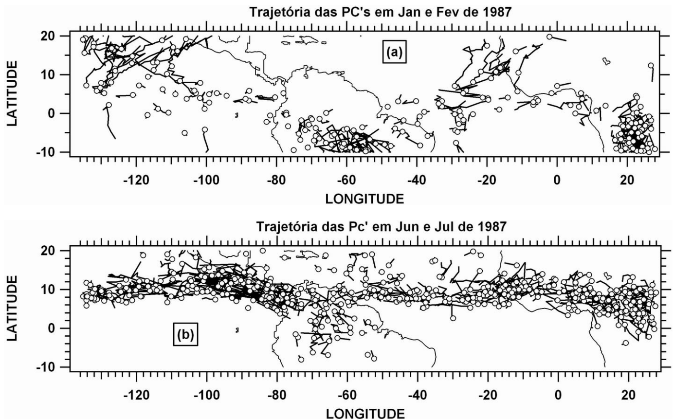
Figura 2: Trajetória das perturbações convectivas (PC) que ocorreram em janeiro e fevereiro de 1987 (a), e, as que ocorreram em junho e julho de 1987 (b), onde o círculo vazio marca a iniciação da PC.
