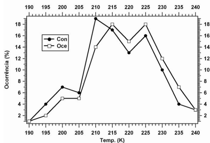
Figura 6: Histograma da temperatura mínima no momento da maturação da perturbação convectiva.
