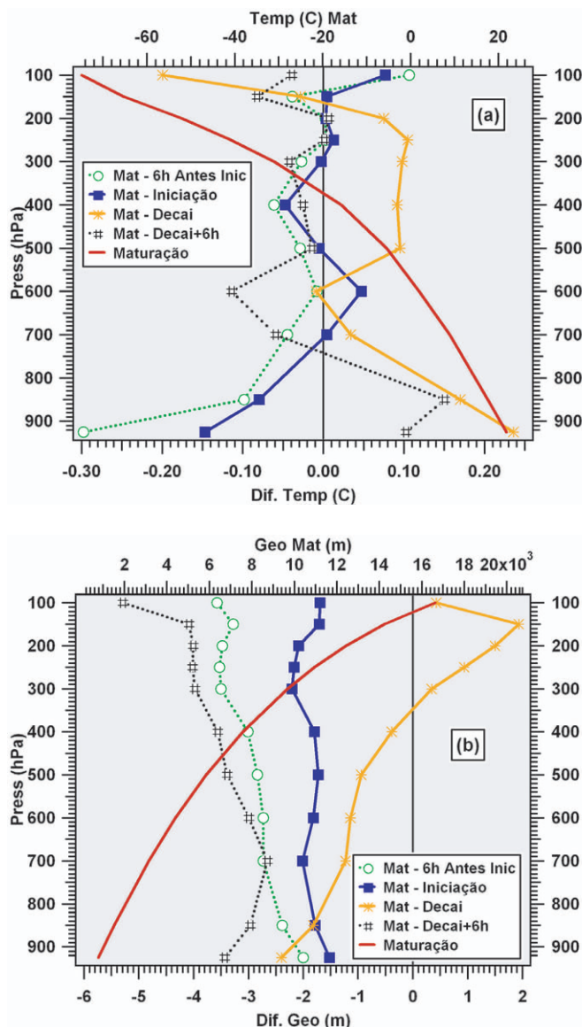
Figura 4: Perfil perturbado da maturação (Mat) e as diferenças entre os perfis perturbados da maturação e os outros momentos do ciclo de vida, onde M-I06 é a diferença entre o perfil perturbado na maturação e seis horas antes da iniciação, M-I é maturação menos iniciação, M-D é maturação menos decaimento, M-D06 é maturação menos seis horas após decaimento, sendo que (a) apresenta a temperatura, (b) o Geopotencial, (c) a umidade e (d) a omega.
