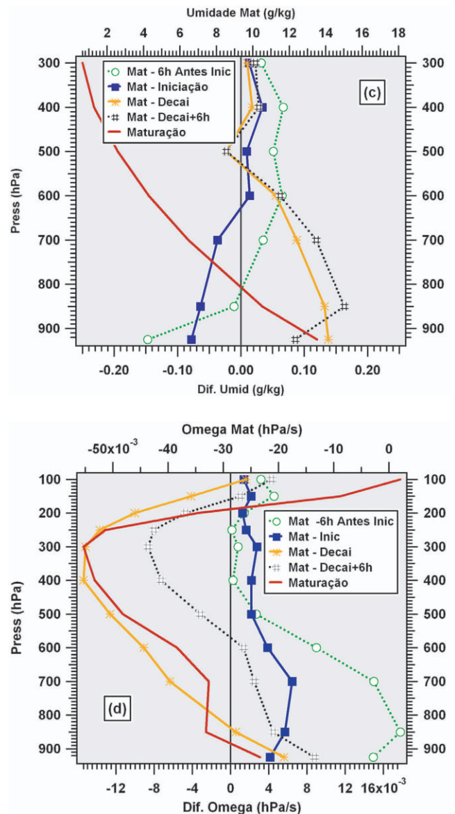
Figura 4: Perfil perturbado da maturação (Mat) e as diferenças entre os perfis perturbados da maturação e os outros momentos do ciclo de vida, onde M-I06 é a diferença entre o perfil perturbado na maturação e seis horas antes da iniciação, M-I é maturação menos iniciação, M-D é maturação menos decaimento, M-D06 é maturação menos seis horas após decaimento, sendo que (a) apresenta a temperatura, (b) o Geopotencial, (c) a umidade e (d) a omega.
