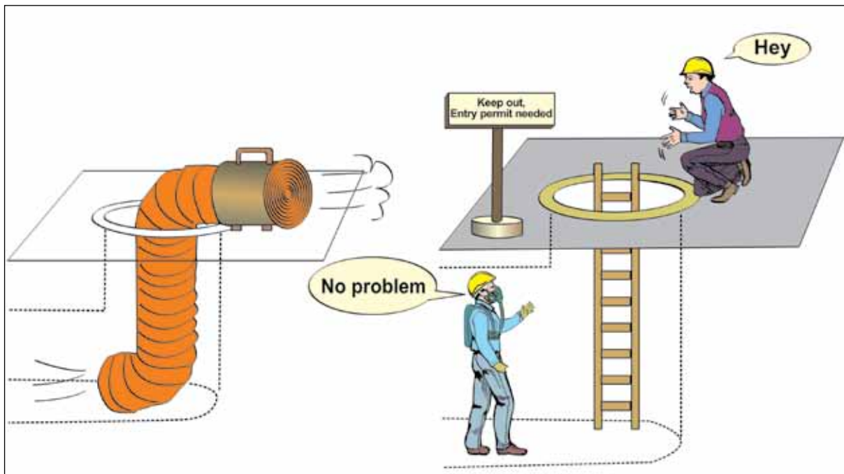
Figura 93b. Antes de entrar em um espaço confinado, certifique-se de que as deficiências de oxigênio e a presença de gases perigosos foram verificadas e que as medidas de controle foram tomadas para que os funcionários trabalhem de forma segura dentro do espaço confinado. Ventilação suficiente do ar no interior é geralmente necessária. Os supervisores e trabalhadores precisam se manter em comunicação durante o trabalho, e as regras sobre o uso de tipos designados de equipamento de proteção pessoal devem ser estritamente seguidas ao trabalhar dentro do espaço confinado.
