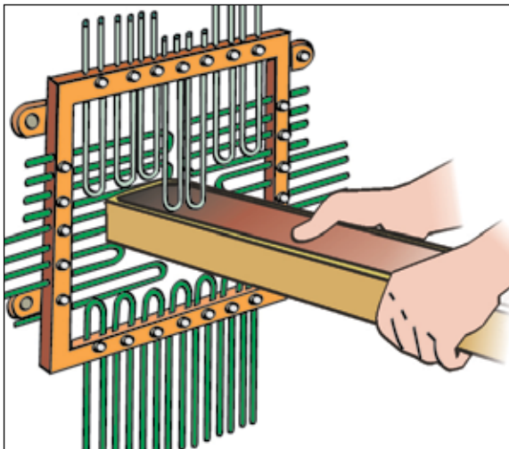
Figura 47a. Uma prensa mecânica com alimentador de êmbolo.
