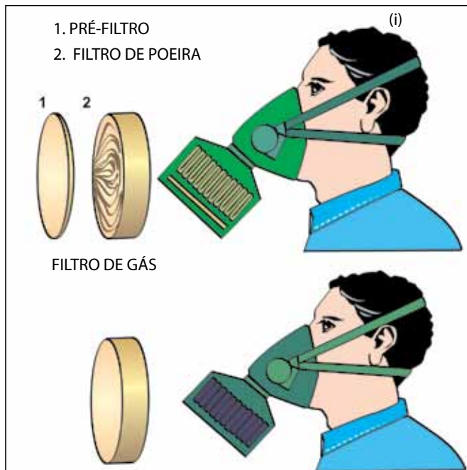
Figura 102a. (i) e (ii) Três tipos de máscaras com filtro. No alto, à esquerda: Com proteção contra partículas conduzidas pelo ar, como, por exemplo, pó de pedra. Abaixo, à esquerda: Com proteção contra gases e fumaça, como, por exemplo, no uso de tintas que contêm solventes. Esse filtro contém carbono ativado. Acima: Com um filtro combinado, contendo tanto filtro de poeira quanto de gás. Essas máscaras são exemplos da proteção respiratória eficaz mais simples. Substitua o filtro quando a respiração se tornar difícil ou quando começar a exalar odor. Faça-o com frequência.
