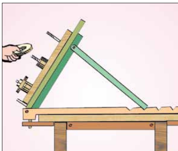
Figura 44c. As fixações que estabilizam as operações muitas vezes podem ser projetadas facilmente.
