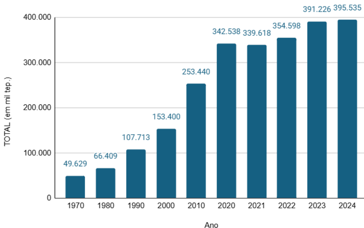
Gráfico 2. Total de energia produzida (em mil tep)
