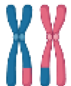
Cromossomo (Recombinante)
