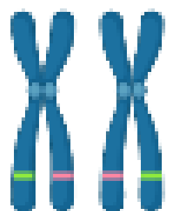
Cromossomo (Heterozigoto)
