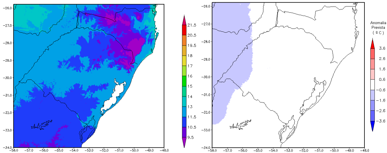
Figura 9. Temp. Mínima Média Climatologia (°C) e Anomalia Prevista maio/2016
