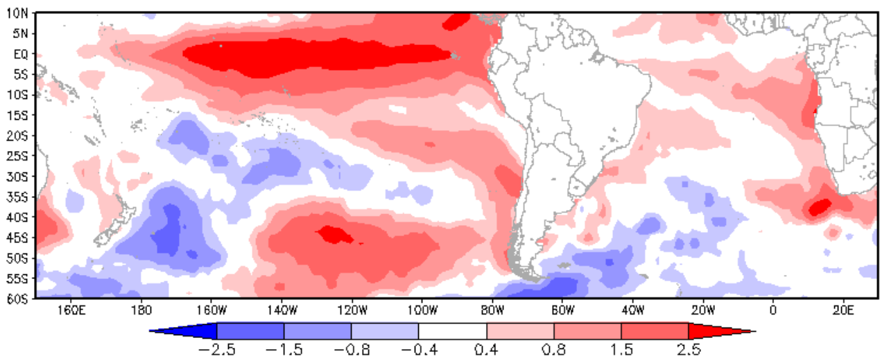
FIGURA 3. Anomalia Mensal de TSM, Janeiro/2016, Fonte: NOAA-CDC/UFPel-CPPMet.
