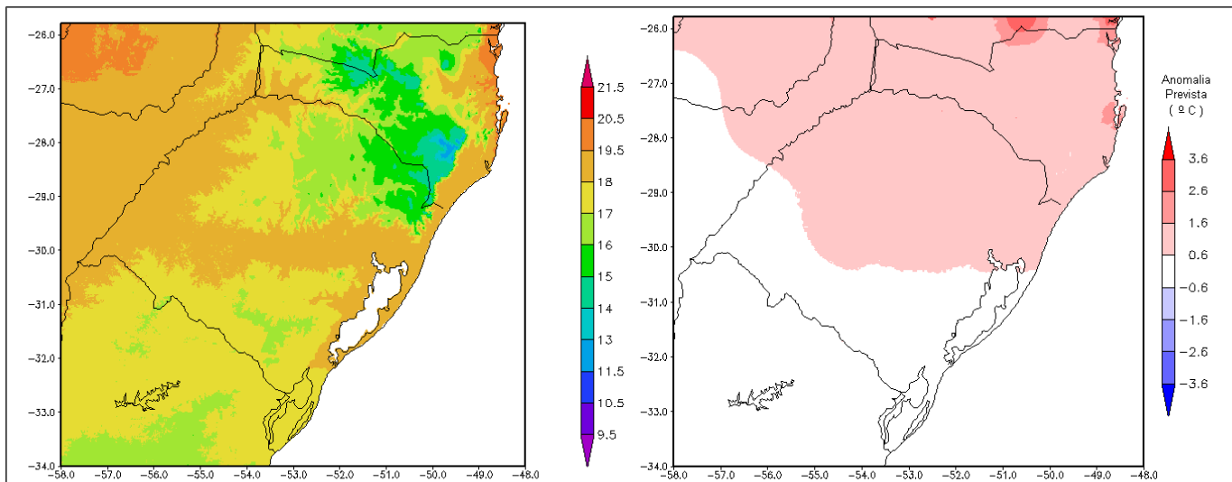
Figura 7. Temp. Mínima Média Climatologia (°C) e Anomalia Prevista março/2016
