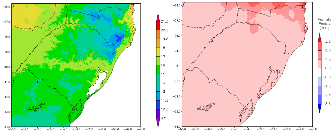
Figura 8. Temp. Mínima Média Climatologia (°C) e Anomalia Prevista abril/2016
