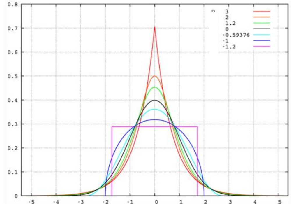
Excesso de curtose
