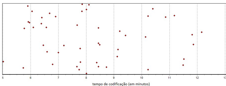
Figura 11. Tempos de codificação (em minutos) de uma função padrão em uma determinada linguagem de programação de 50 programadores experientes.
